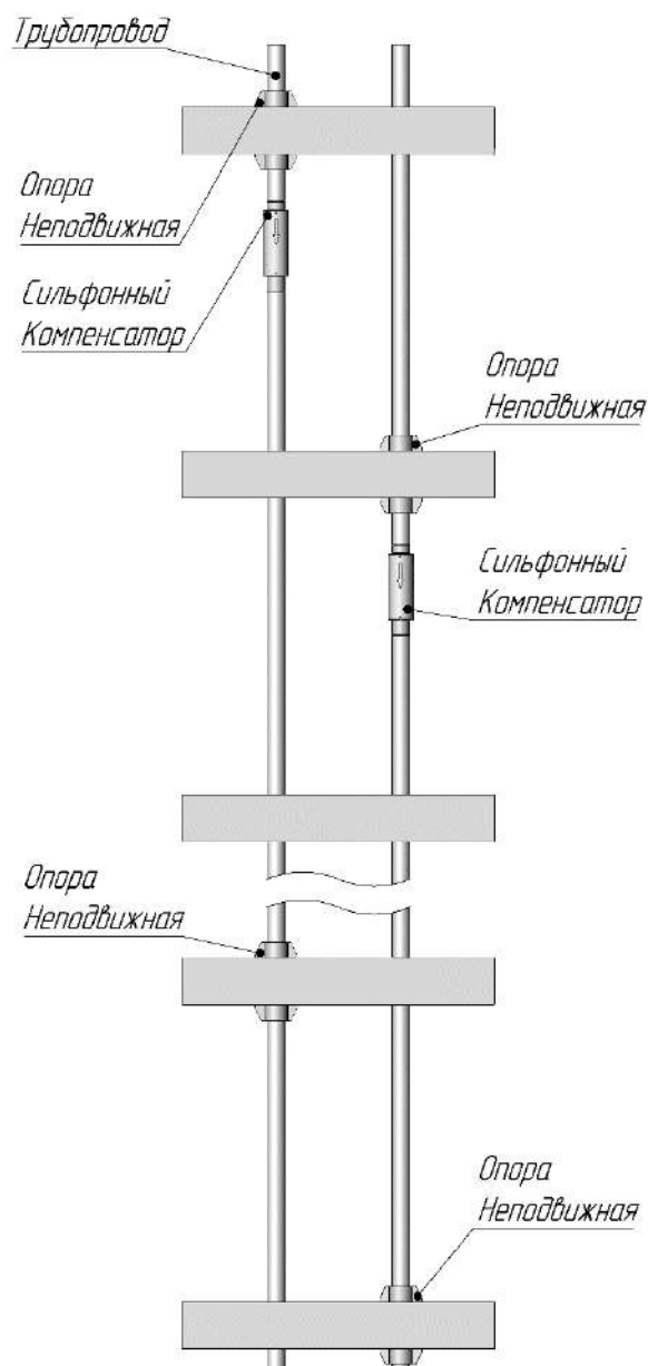
Рис.15.2 Схема разнесения неподвижных опор и сильфонных компенсаторов по этажам.
