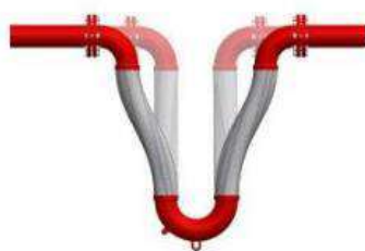
⚙ U-flex: расширение
