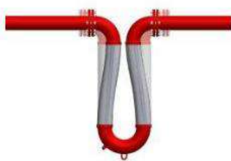
⚙ U-flex: сжатие
